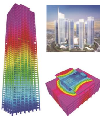
Omnix Tower (UAE)
